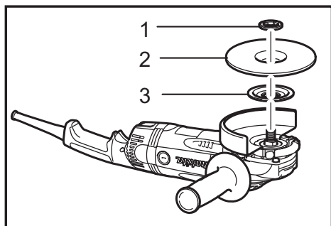
► 1. Contratuercia 2. Disco para esmerilar de centro hundido / multidisco 3. Brida interior
