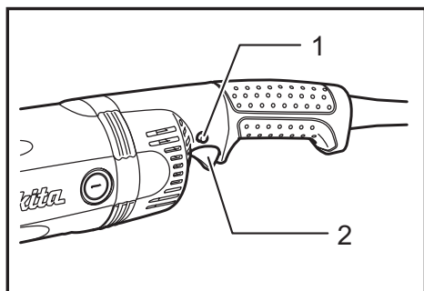
► 1. Bouton de verrouillage / Bouton de sécurité 2. Gâchette
