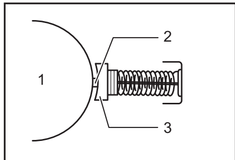
► 1. Conmutador 2. Punta de aislante 3. Escobilla de carbón
