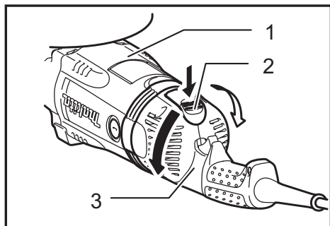
► 1. Alojamiento del motor 2. Botón de bloqueo 3. Mango
