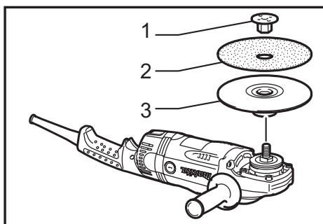
► 1. Contratuercia 2. Disco abrasivo 3. Plato de goma
