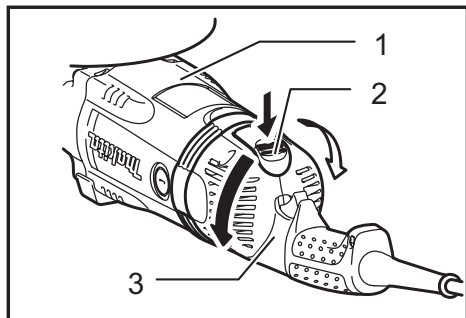
► 1. Boîtier du moteur 2. Bouton de verrouillage 3. Manche
