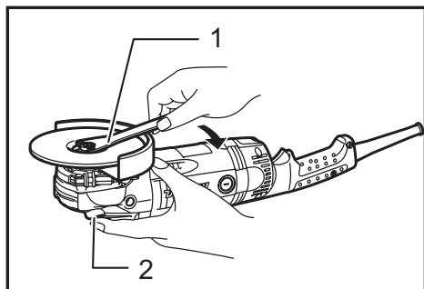
► 1. Llave de tuerca 2. Bloqueo del eje
