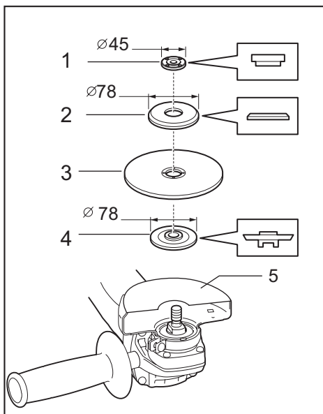
► 1. Contratuerca 2. Brida exterior 78 3. Disco de corte abrasivo / Disco de diamante 4. Brida interior 78 5. Protector de disco para disco de corte abrasivo / disco de diamante
