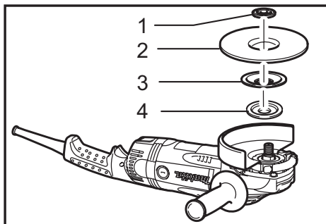
► 1. Contratuercia 2. Disco flexible 3. Plato de goma 4. Brida interior
